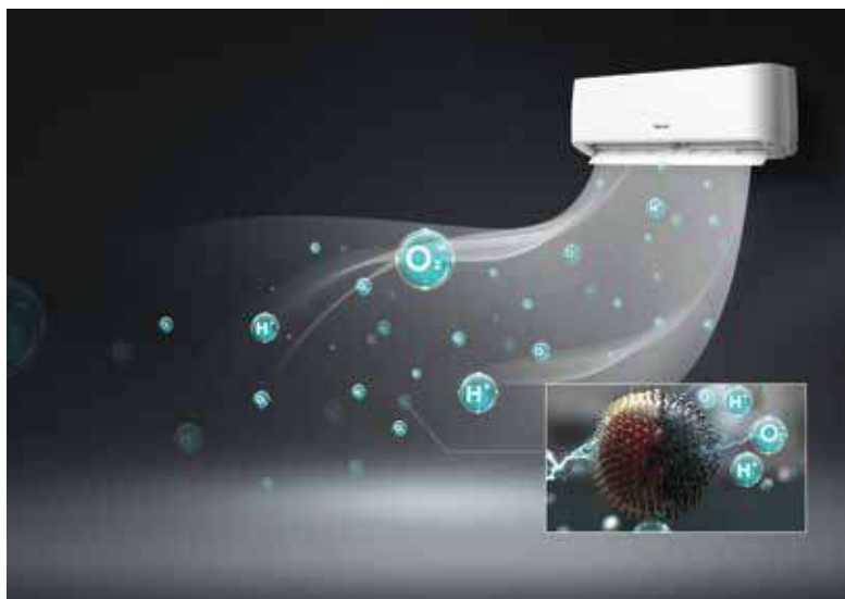
Ionizace
